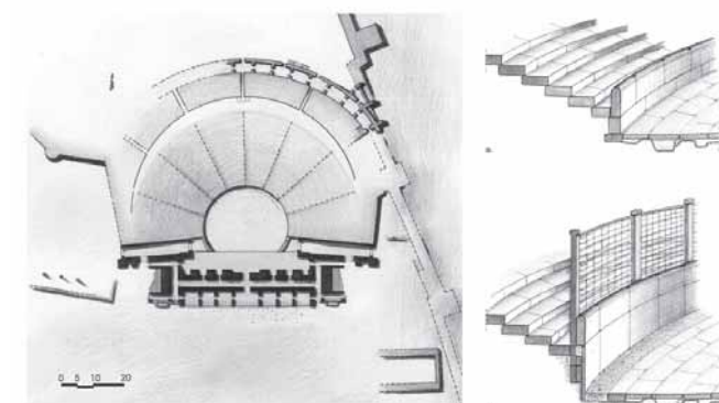
Εικ. 4. Θέατρο Φιλίππων: Πρώτη φάση αρένας, κατά την οποία υπάρχει παράλληλη χρήση θεάτρου και αρένας.
